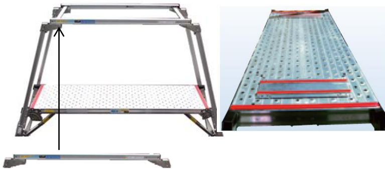
妻側が一体になったセーフティガード
