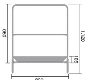
妻面手摺(固定) 6kg
