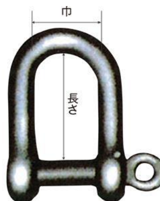
捻込シャックル 規格寸法
