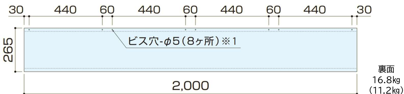
正面図
