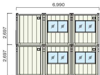
立面図
