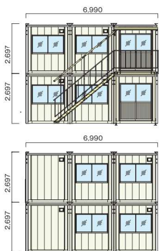
立面図
