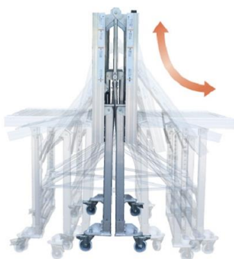
折畳式でコンパクト収納 エレベーターへの搭載も可能
